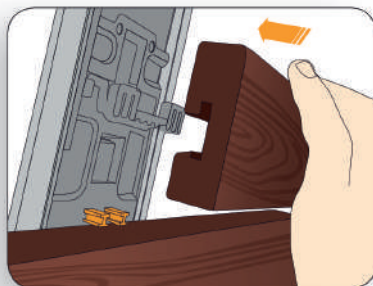
5 : Pose de la lame suivante
